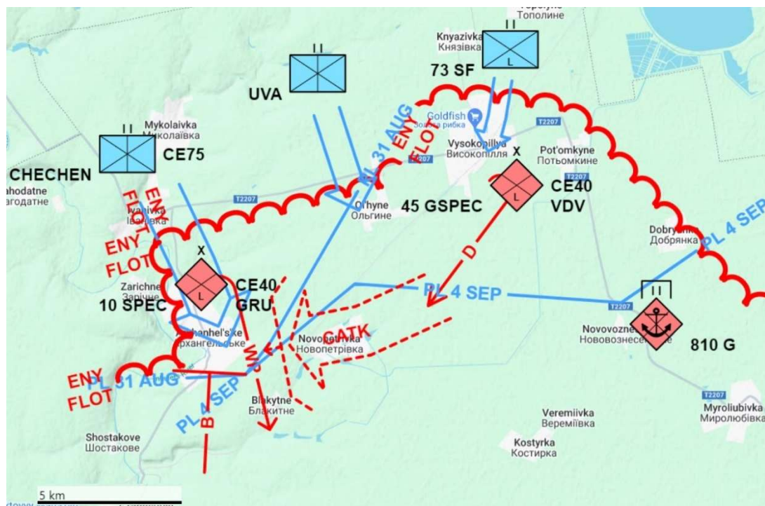
26. ábra: Az Arhengelszke és Vyszokopillija környéki műveletek vázlatja 2022. szeptember első napjaiban. A szerző saját munkája.
