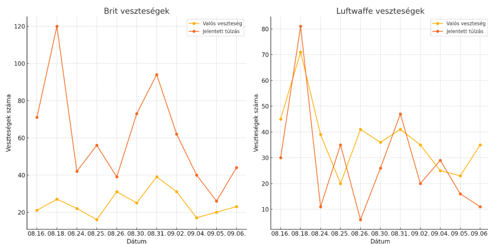
30. ábra A Luftwaffe és a RAF valós és lejelentett veszteségeinek szemléltetése
