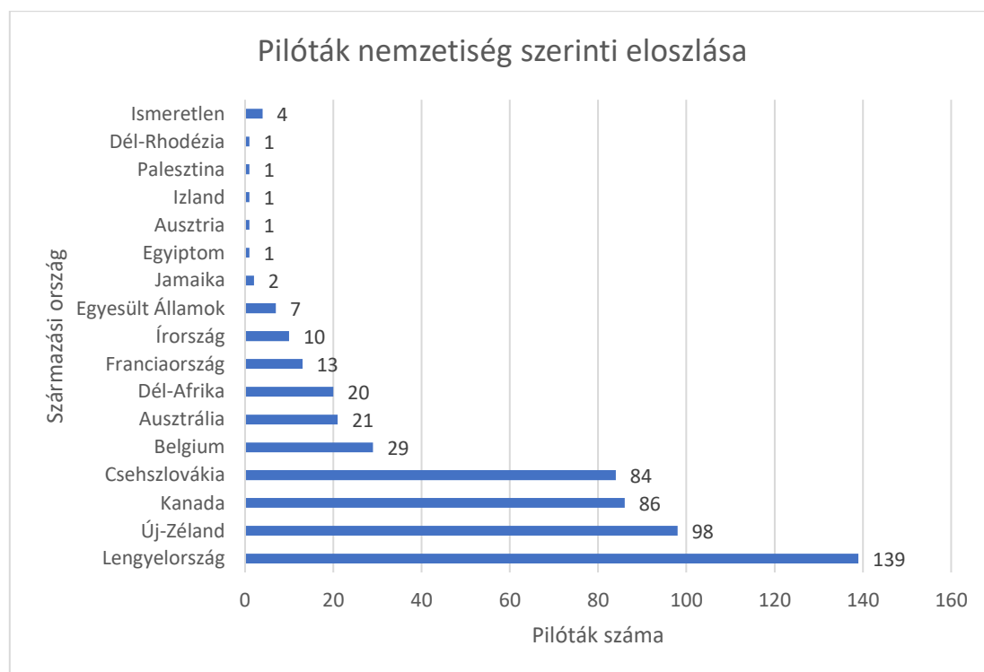
13. ábra: a nem brit pilóták nemzetiség szerinti eloszlása Patrick Bishop könyve szerint 124
